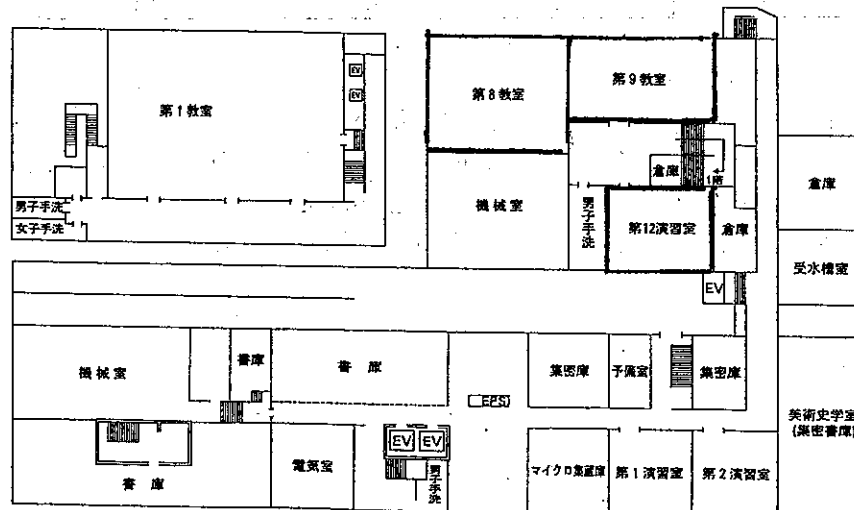
地階平面図
