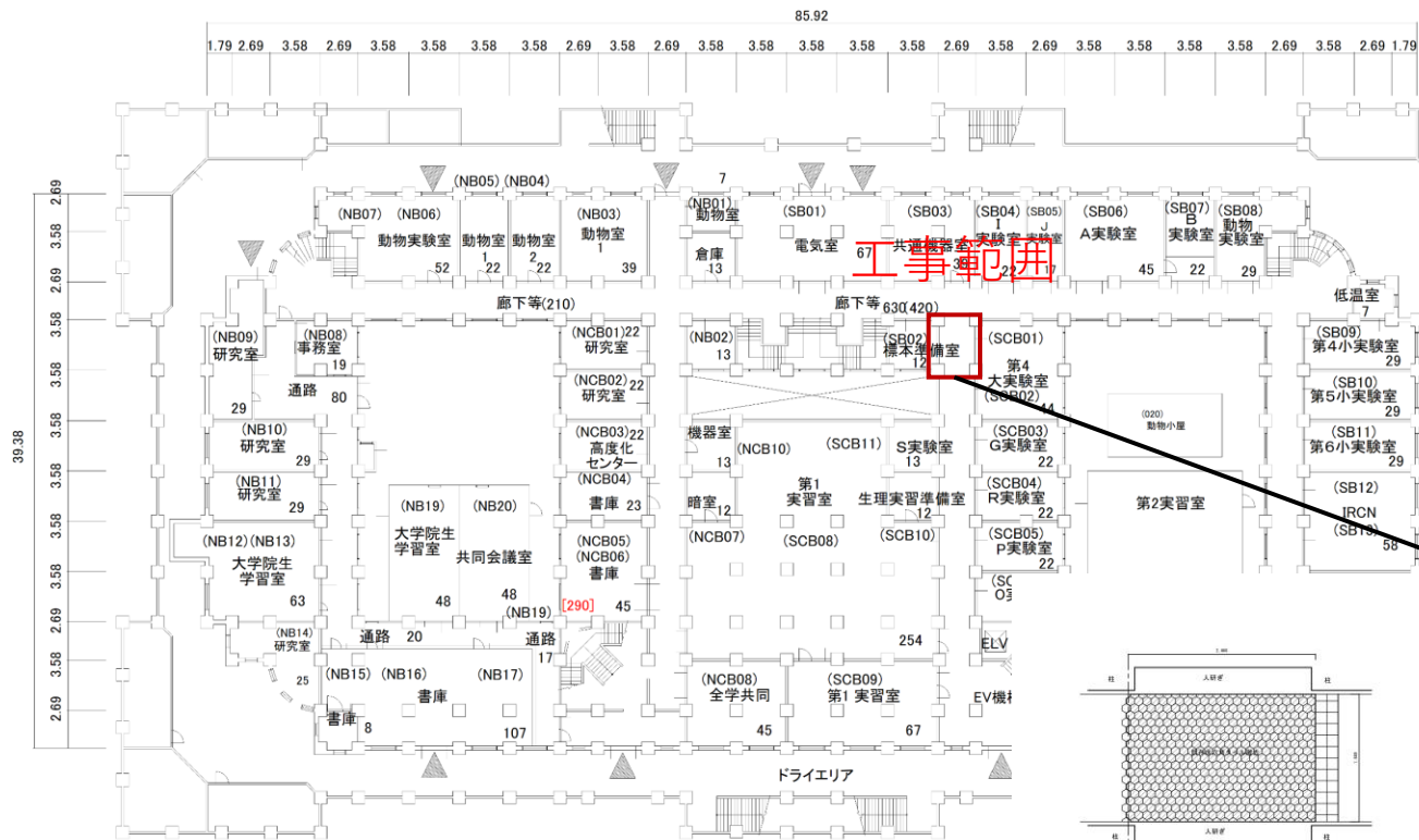
医学部1号館地階平面図 2,721m 2 S=
